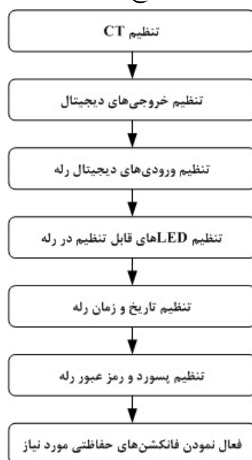
شکل 8-1: روندنمای تنظیمات اولیه رله ثانویه
