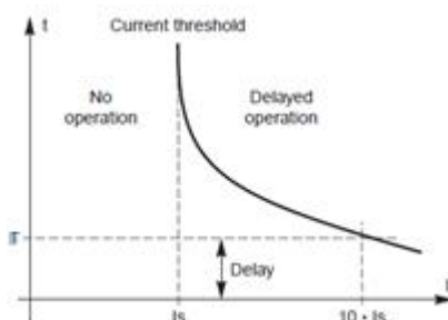
شکل 2-5؛ منحنی جریان-زمان معکوس
