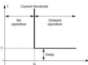
شکل 1-5؛ منحنی زمان معین
